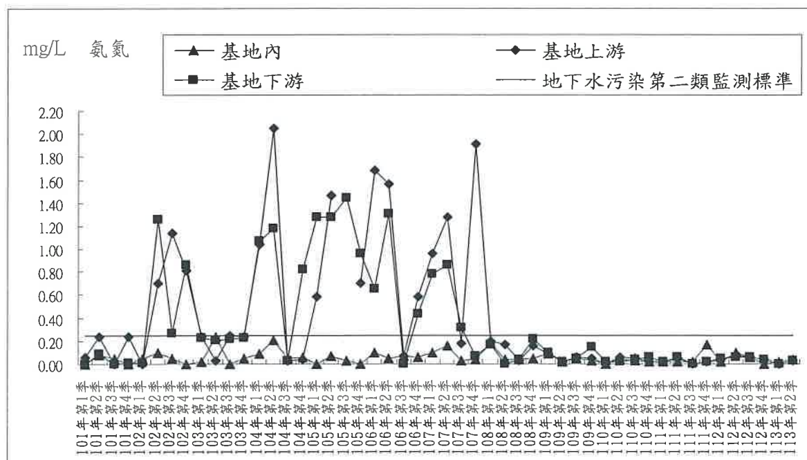
圖 2.3-12 地下水質氮氮監測結果
