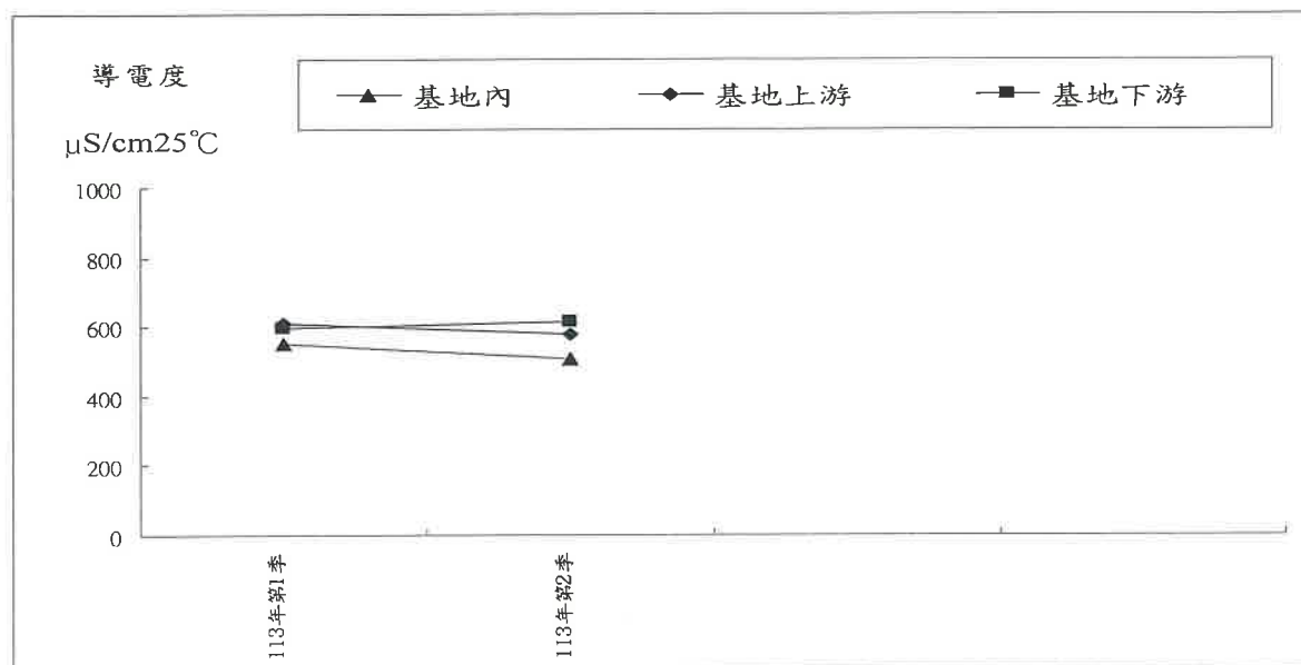
圖 2.3-15 地下水質導電度監測結果
