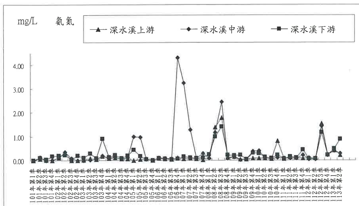
圖 2.3-4 地面水質氮氮監測結果
