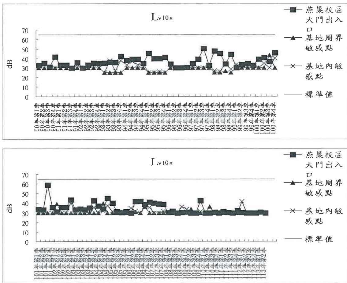
圖 2.2-6 振動 L_{v10dB} 監測結果
