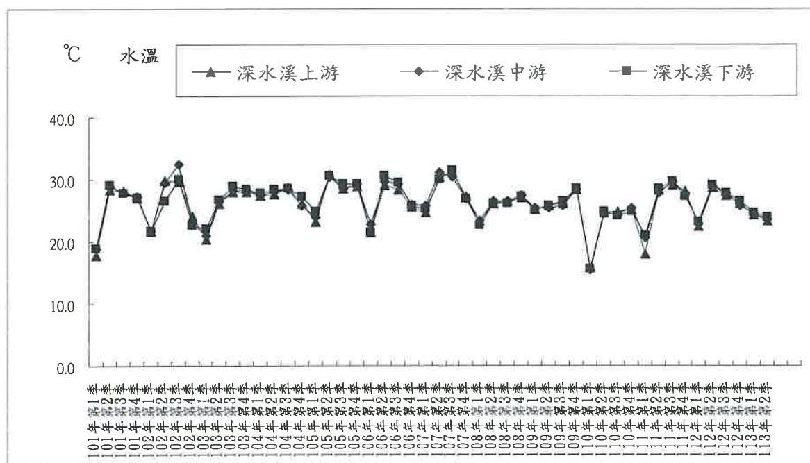
圖 2.3-2 地面水質水溫監測結果
