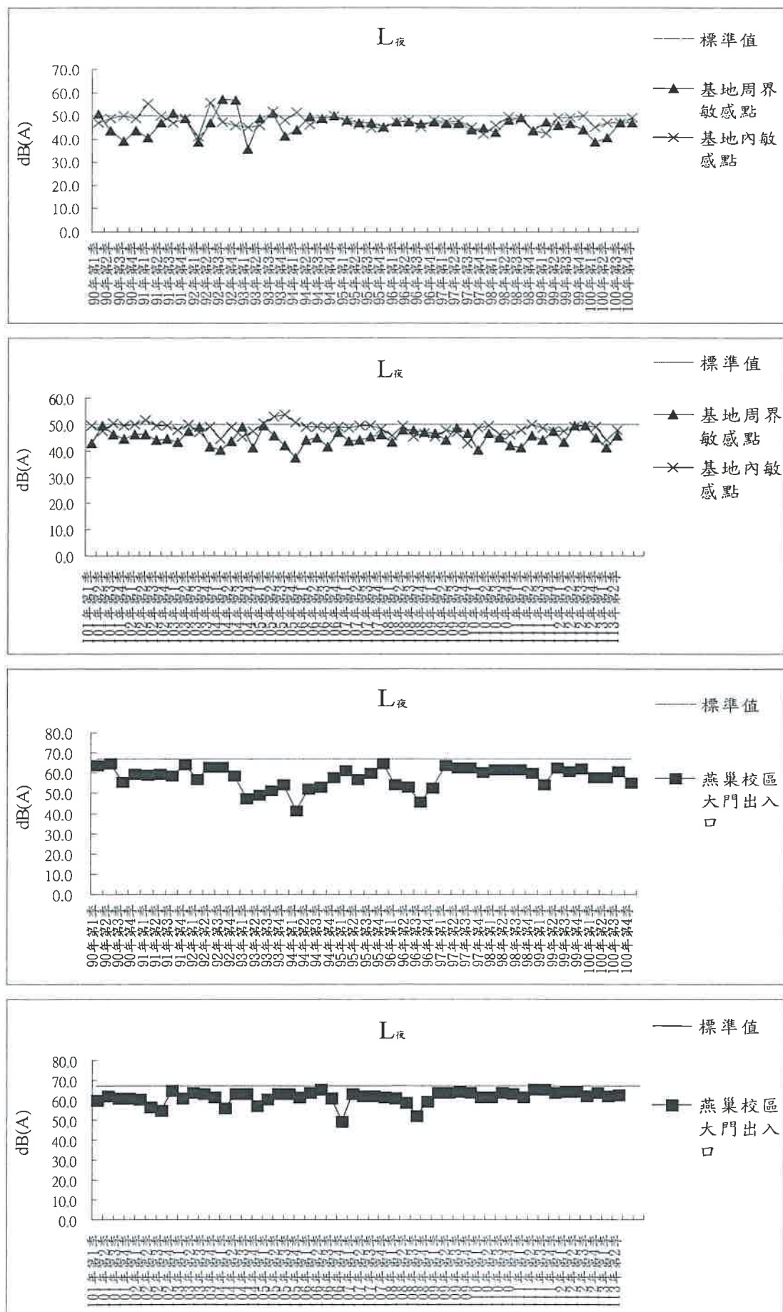
圖 2.2-3 噪音 L_{夜} 監測結果
