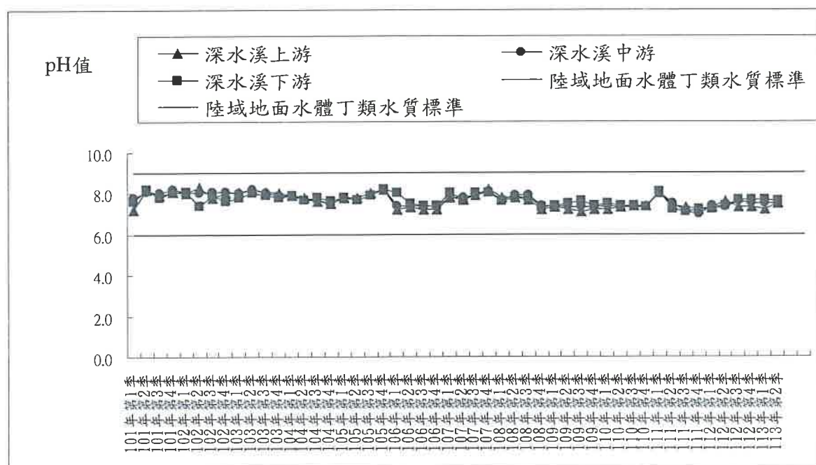
圖 2.3-1 地面水質 pH 值監測結果
