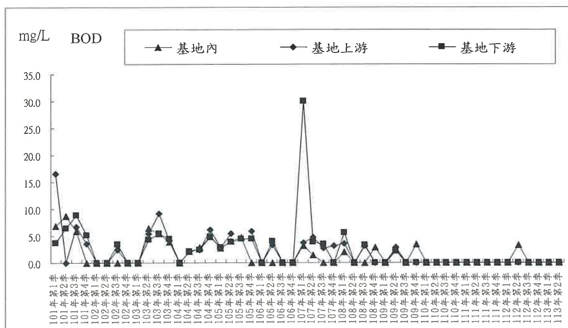
圖 2.3-13 地下水質 BOD 監測結果
