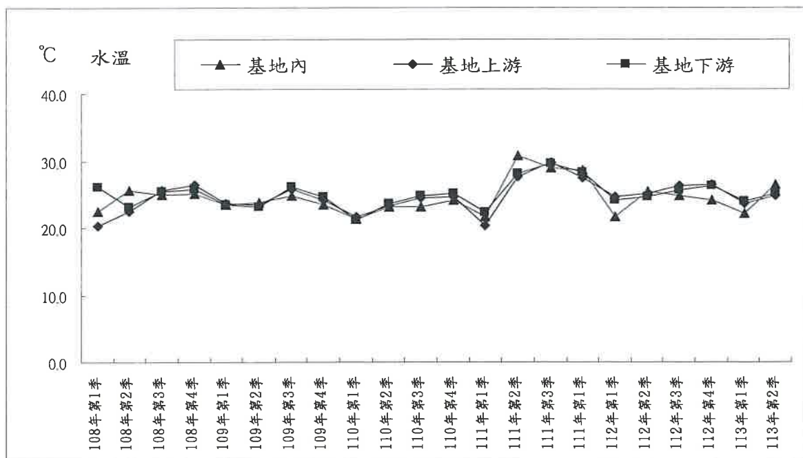
圖 2.3-17 地下水質水溫監測結果
