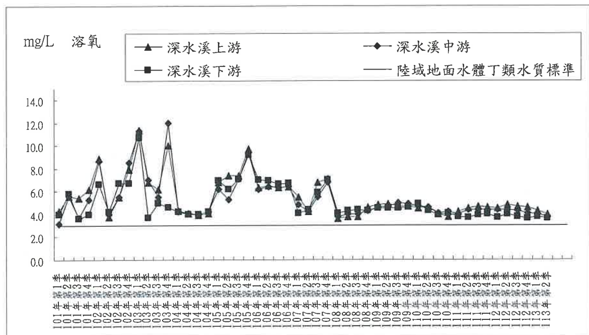
圖 2.3-6 地面水質溶氧監測結果
