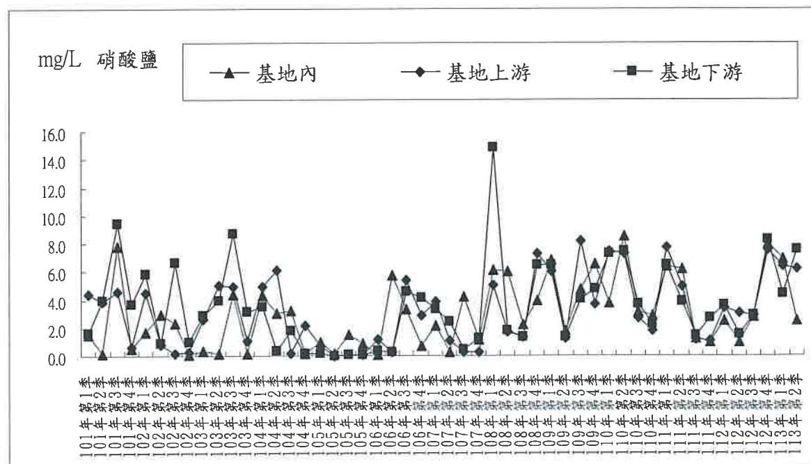
圖 2.3-16 地下水質硝酸鹽監測結果
