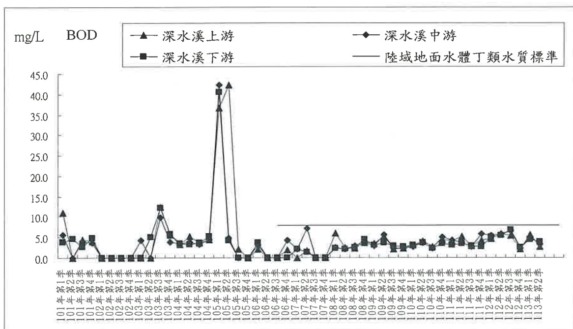
圖 2.3-5 地面水質 BOD 監測結果
