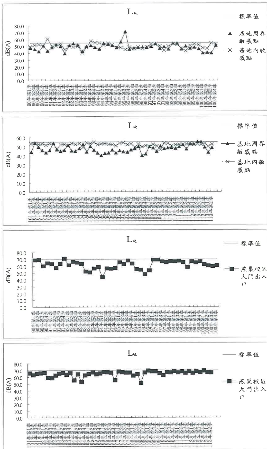
圖 2.2-2 噪音 L_{晚} 監測結果
