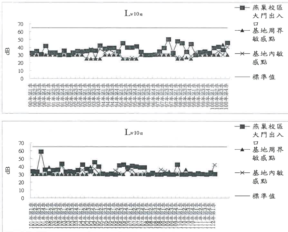
圖 2.2-6 振動 L_{v10} 監測結果
