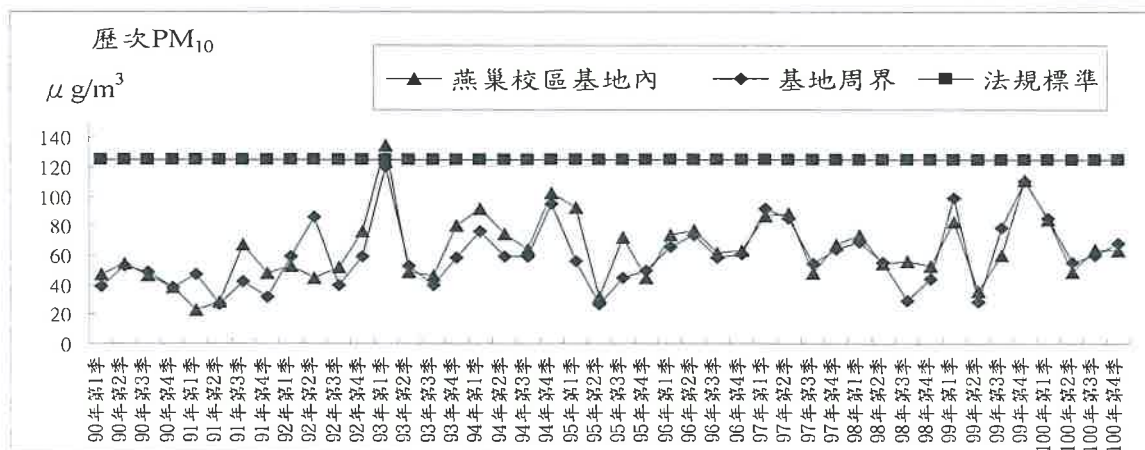
圖 2.1-1 空氣品質監測結果
