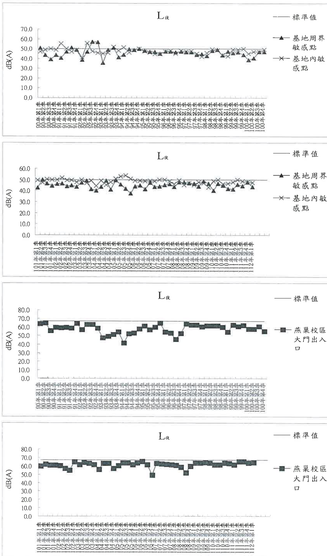
圖 2.2-3 噪音 L 夜 監測結果
