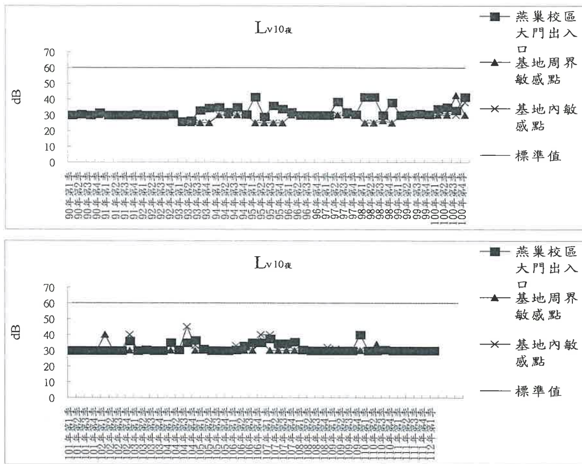
圖 2.2-7 振動 L_{v10} 夜監測結果
