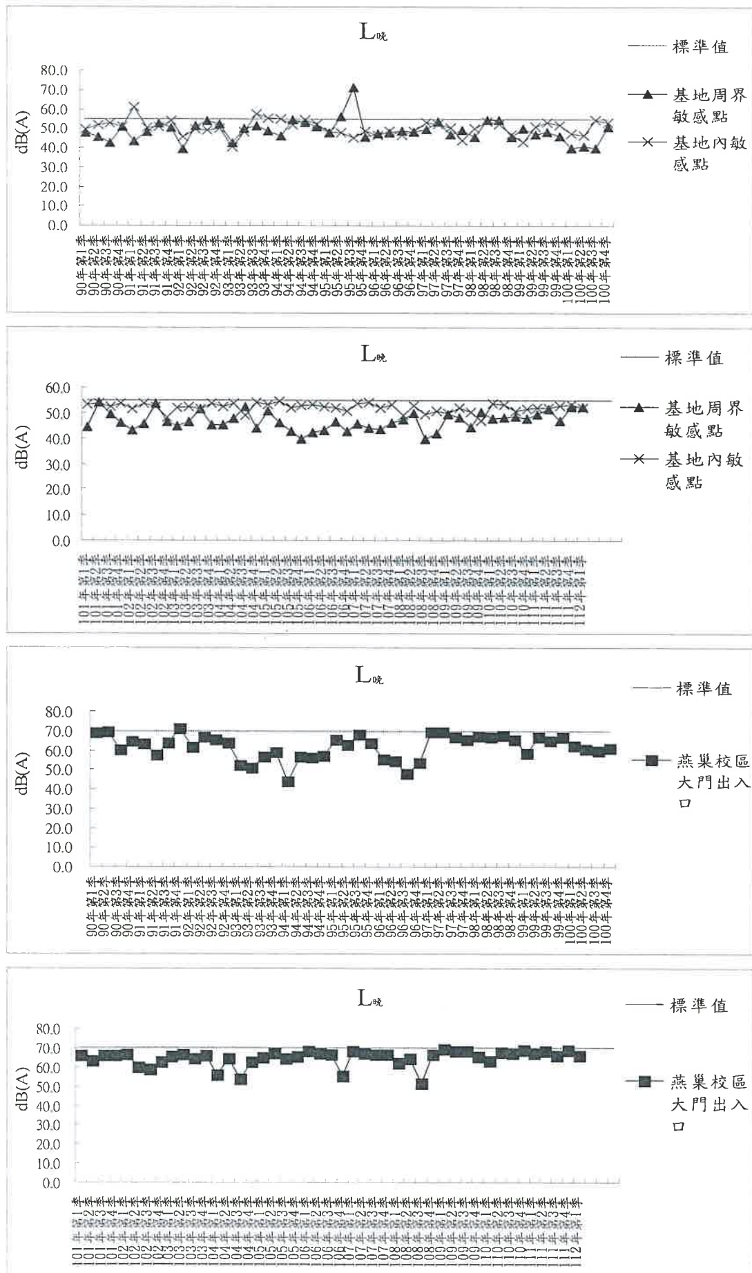
圖 2.2-2 噪音 L_{晚} 監測結果
