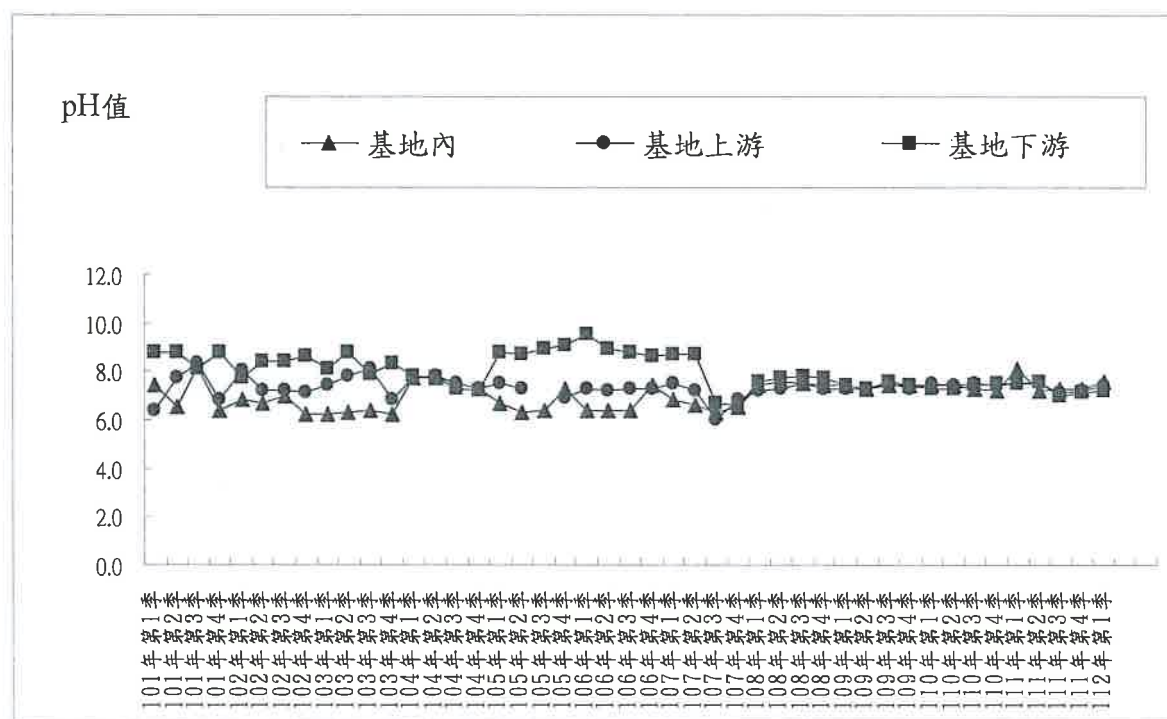
圖 2.3-10 地下水質 pH 值監測結果
