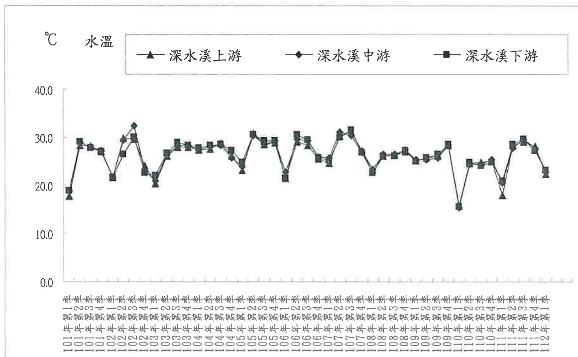
圖 2.3-2 地面水質水溫監測結果
