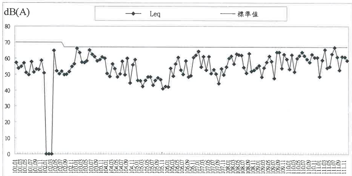
圖 2.2-4 營建噪音 L_{eq} 監測結果
