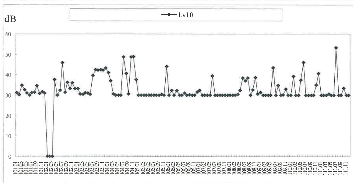
圖 2.2-8 營建振動 L_{v10} 監測結果
