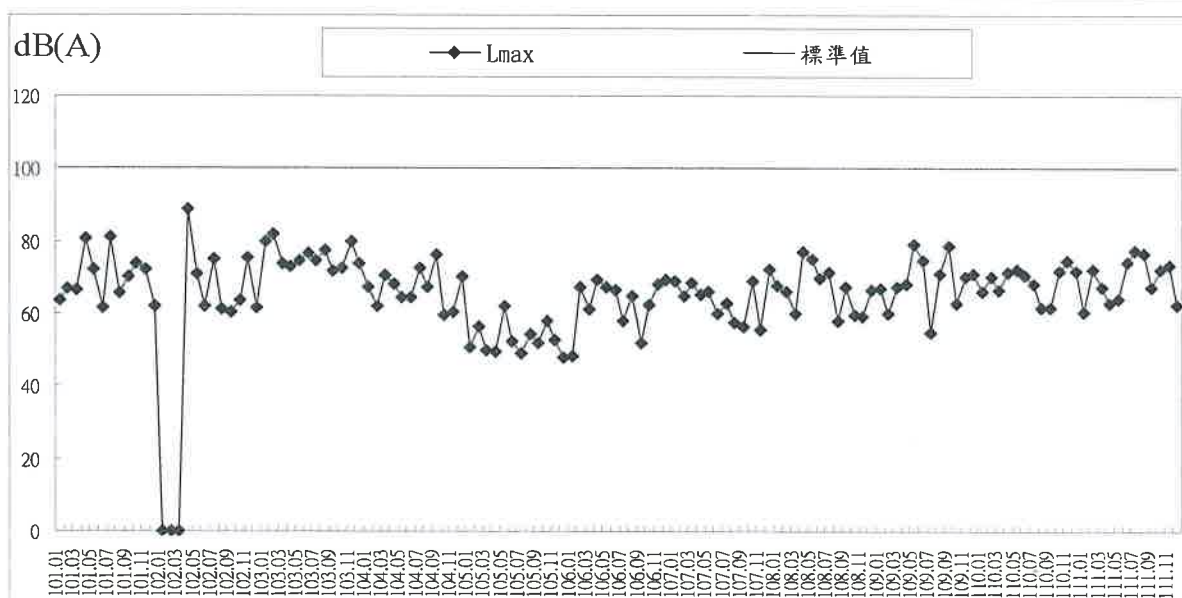
圖 2.2-5 營建噪音 L_{max} 監測結果
